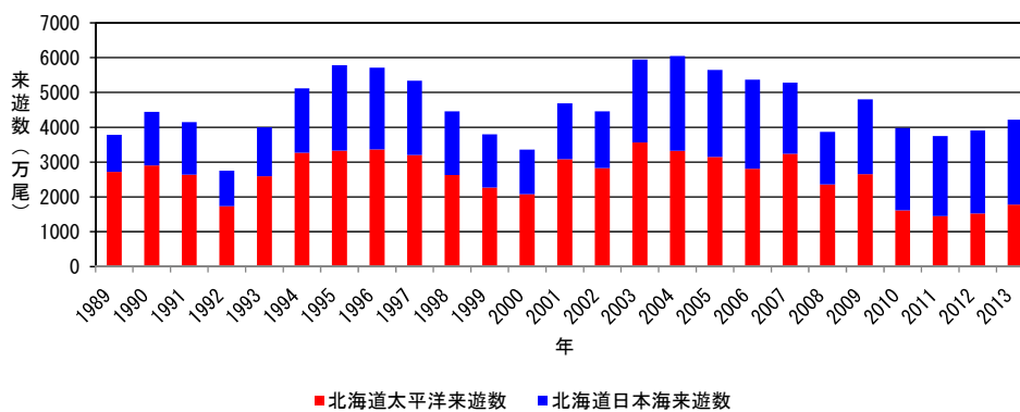
図2. 8月1日～1月31日までのサケ北海道太平洋および日本海来遊数(累計値). 2013年は速報値.
