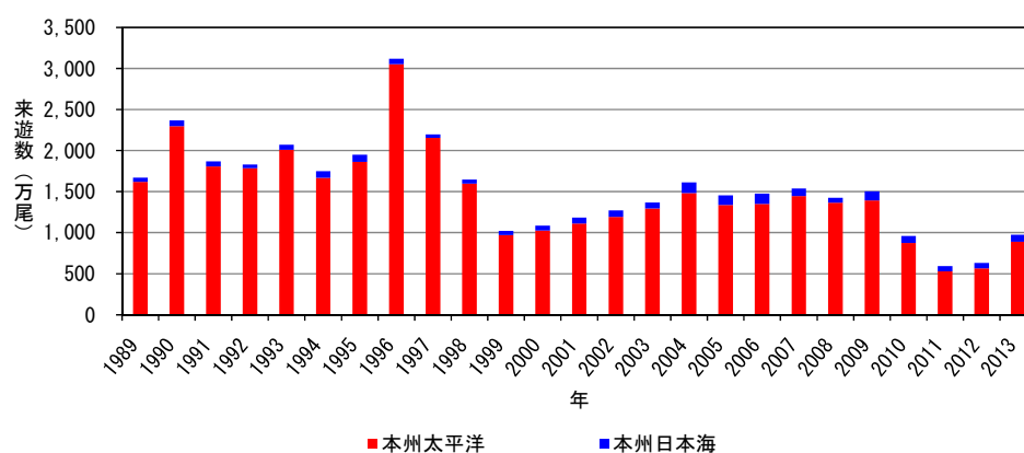
図3. 8月1日～1月31日までのサケ本州来遊数(累計値). 2013年は速報値.
