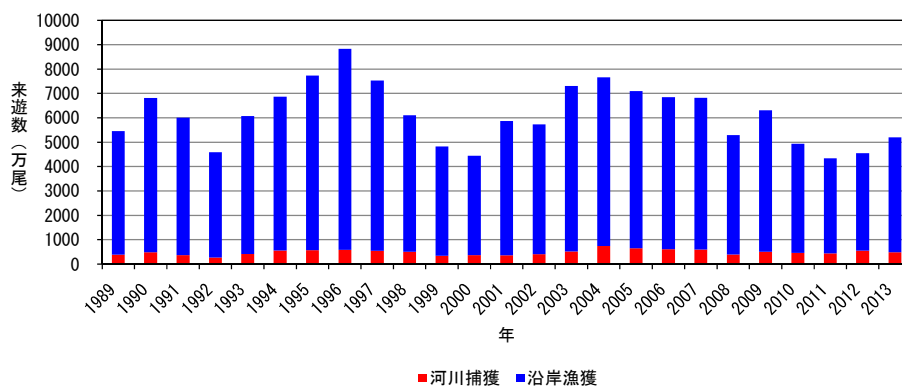
図 1. 8 月 1 日～1 月 31 日までのサケ全国来遊数 (累計値) . 2013 年は速報値.
